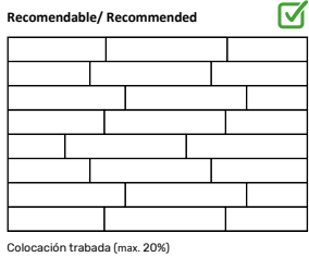
Colocación trabada (máx. 20%)
